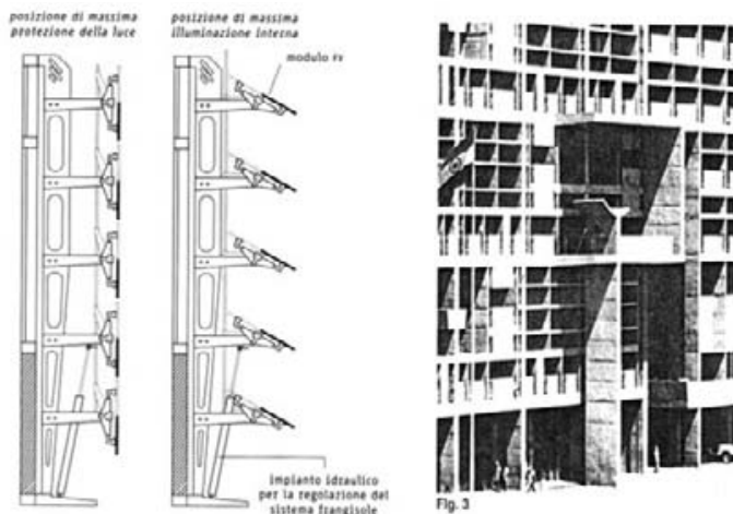
Esempio di schermo per il controllo dell'irraggiamento solare e contestualmente inserimento di pannelli di fotovoltaico
