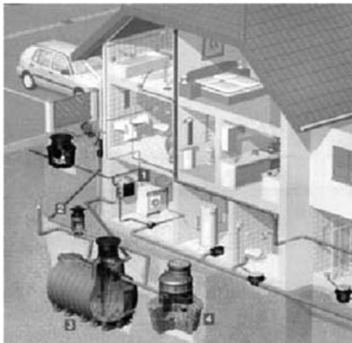
(1) centralina per il reintegro; (2) filtro; (3) serbatoio di raccolta; (4) sistema di pompaggio
