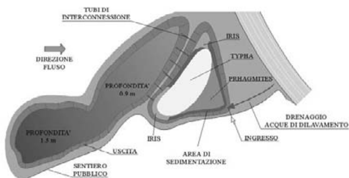
Esempio di sistema di fitodepurazione per il trattamento del runhoff stradale
