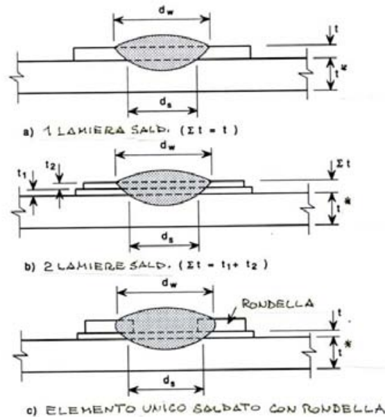
Figura C4.2.35 – Saldature a bottone
