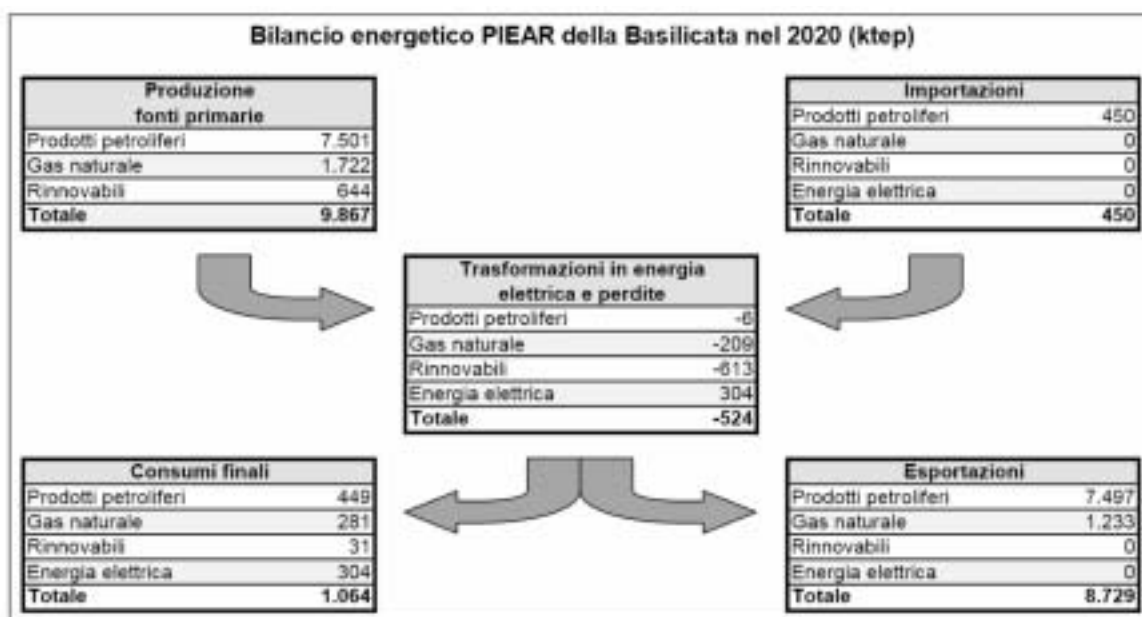
Fig. 3" - K: Schema di sintesi del bilancio energetico PIEAR della Basilicata nel 2020 41 (fonte: Regione Basilicata).
