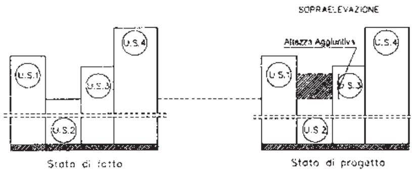
Esempio di intervento su unità strutturale 2
