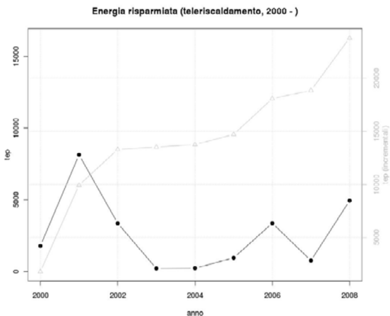
Figura 8.12: Teleriscaldamento
