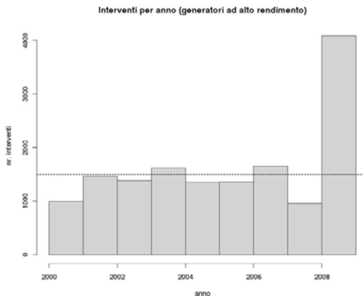
Figura 5.1: Gli interventi di sostituzione di generatori di calore sono spesso parte di interventi integrati che coinvolgono più tecnologie (abbiamo 9649 interventi singoli e 5214 interventi integrati di cui 84% prioritari, che coinvolgono cioè la generazione di energie rinnovabili). Il grafico riporta il numero totale di interventi (incluso quindi gli interventi integrati). La linea tratteggiata orizzontale (di ordinata pari a 1500) rappresenta l'obiettivo di piano in termini di numero di interventi.
