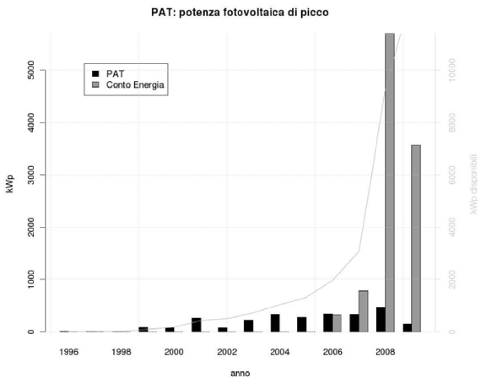
Figura A.1: I contributi per la costruzione degli impianti fotovoltaici sono di tipo provinciale (dagli anni 90) e nazionale (il "Conto energia", negli ultimi anni). La scala di destra corrisponde al totale dell'energia di picco installata riportata in linea continua.
