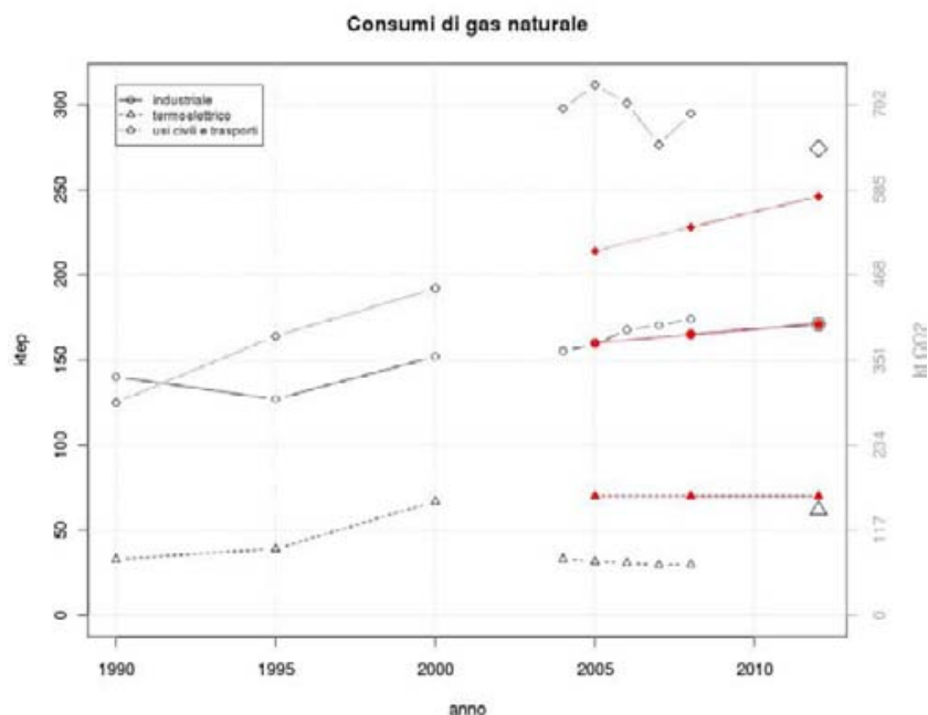
Figura 1.2: L'analisi dei consumi suddivisi per settori mostra che l'utilizzo per usi civili è significativamente maggiore di quanto preventivato. Il grafico presenta una discontinuità dovuta alle diverse modalità di rendicontazione nei periodi considerati. I dati fino al 2000 sono corretti per l'attribuzione al settore termoelettrico. Quelli del 2004 e successivi, basati sui bollettini DGERM, non attribuiscono al settore termoelettrico i consumi collegati agli impianti di cogenerazione (che appaiono invece negli usi civili). I dati di previsione PEAP sono basati sul primo tipo di rendicontazione. La produzione di energia elettrica da impianti di cogenerazione è riportata in Figura 3.2.
