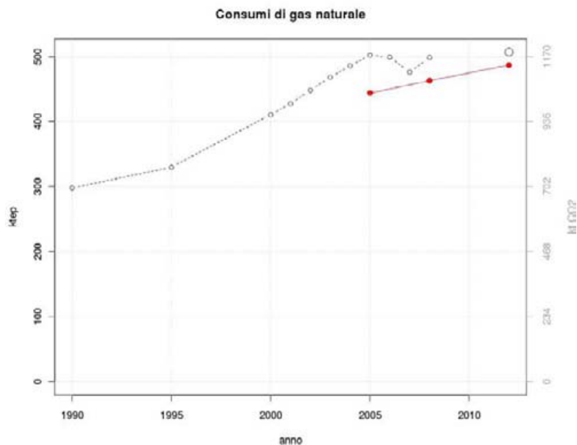
Figura 1.1: I consumi di gas naturale, espressi in migliaia di tep (ktep) per un più facile confronto del contributo relativo delle diverse fonti energetiche. I dischi collegati con linea continua rappresentano la stima proposta nel piano energetico per lo scenario tendenziale ( business as usual ), mentre il cerchio (vuoto) più grande rappresenta lo scenario ipotizzato di risparmio energetico. I consumi attuali sono minori di quanto previsto al 2012 dallo scenario di risparmio energetico di un quantitativo di 8 ktep.
