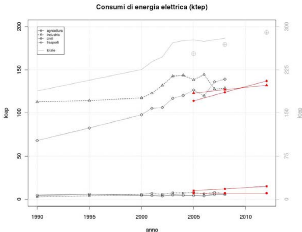
Figura 3.1: L'andamento complessivo dei consumi (linea continua grigia e scala di destra), pur essendo superiore alle previsioni di piano (simbolo bersaglio) sembra compatibile con il raggiungimento degli obiettivi di piano al 2012. La discrepanza maggiore riscontrata è nel settore degli usi civili, il fabbisogno del quale è significativamente maggiore di quanto previsto (+15 ktep).
