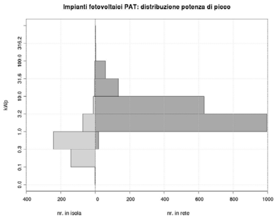
Figura A.2: Sono attualmente in funzione 1846 impianti in rete e 479 in isola, con una potenza rispettivamente di 12413 kWp e 553 kWp per un totale di 12966 kWp.
