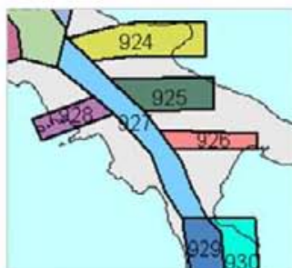
Zonazione Sismogenetica ZS 9 (da AA.VV. ING, 2004)
